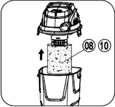
Montaje del filtro de esponja y bolsa de tela
