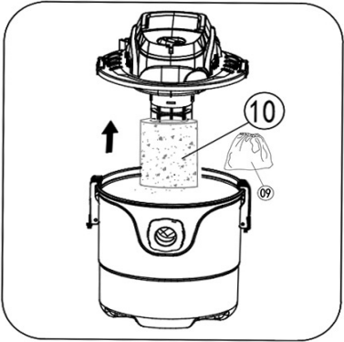
Montaje del filtro de esponja y bolsa de tela
